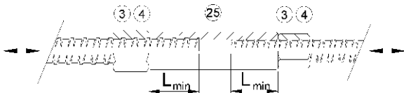
Bild 10 Muffenstoß - Spanschloß Ø12 - 50
