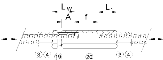
Bild 10 Muffenstoß - Spanschloß Ø12 - 50
