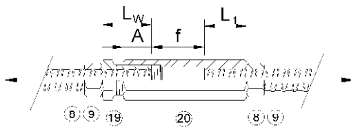
Bild 5 Muffenstoß - Spanschloß Ø12 - 50
