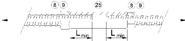
Bild 5 Muffenstoß - Spanschloß Ø12 - 50
