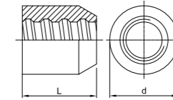
Anschweißstück welding bolt
